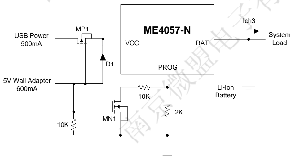
图5：交流适配器与 USB 电源的组合
